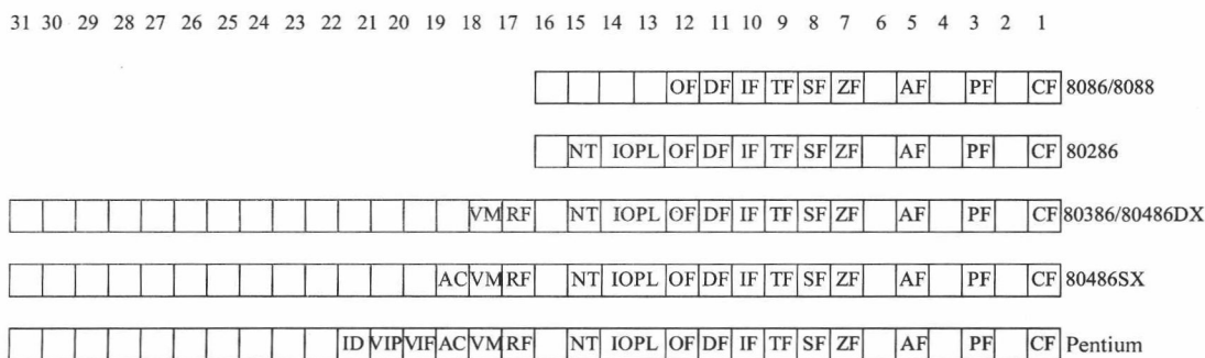
图 1.4 标志寄存器
