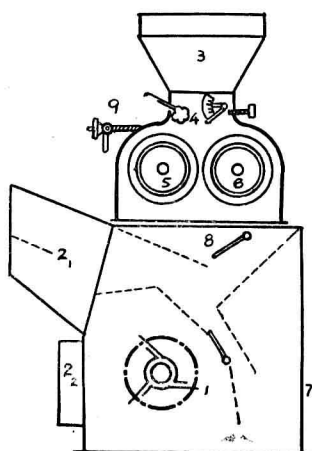
图8 跃进牌胶輥磨谷机结构
