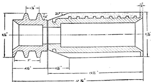
图 5 横式一节砂輥米輥筒图
