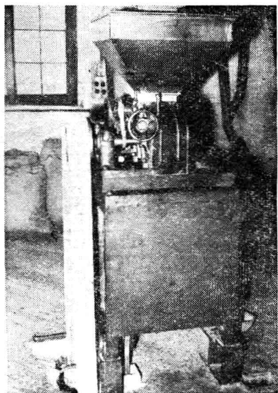
图 7 跃进牌胶輥礱谷机
