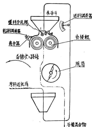
图9 跃进牌磨谷机工艺路线
