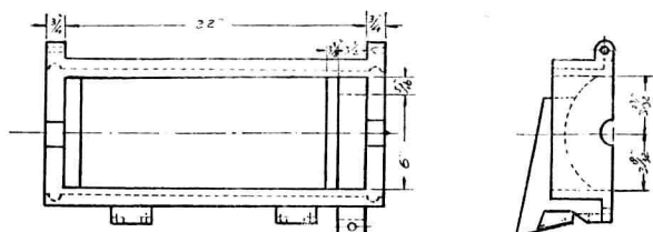
图 2 横式二节砂辊米机的方箱
