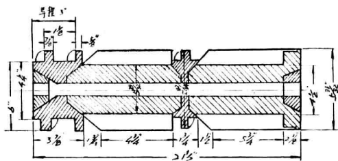
图4 横式二节砂辊米机辊筒的剖面图
