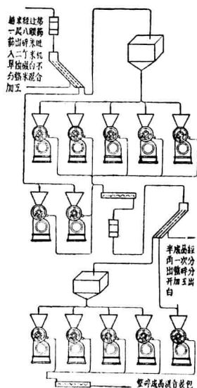
图6 整碎米分粒加工的 工艺流程
