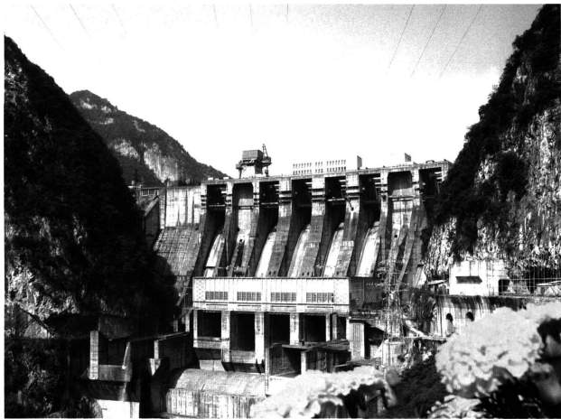
乌江发电厂 (本刊图片资料)
