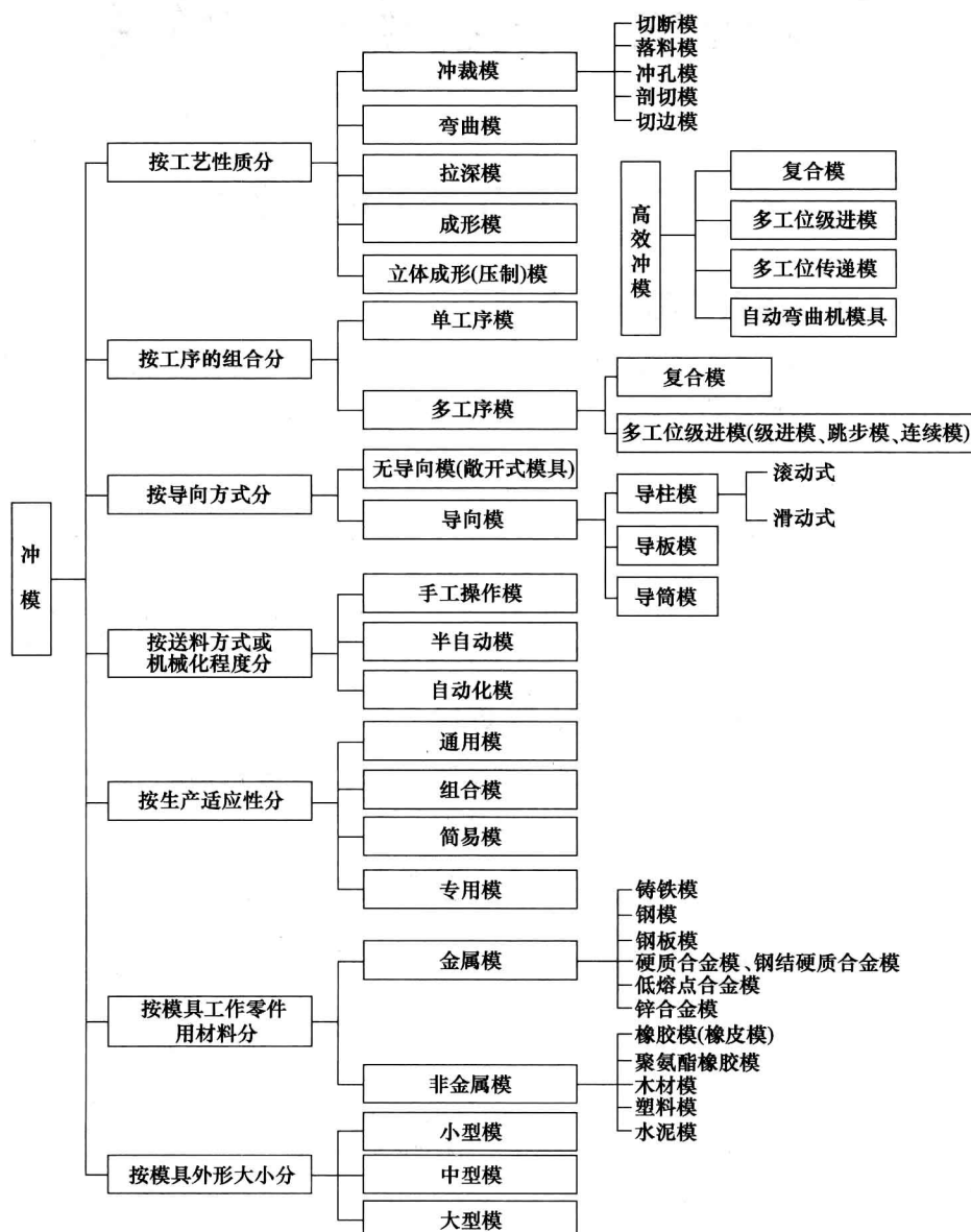
图 1-1 冲模的分类
