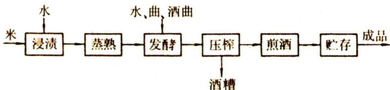
● 黄酒生产流程
