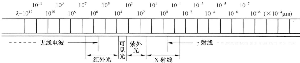
图 1-2 电磁波谱
