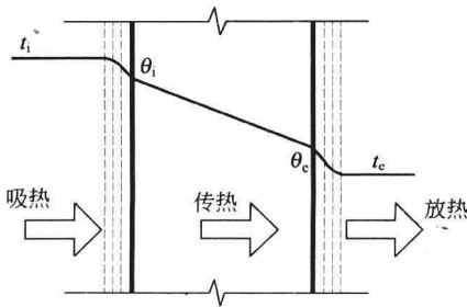
图 14-3 围护结构的传热过程
