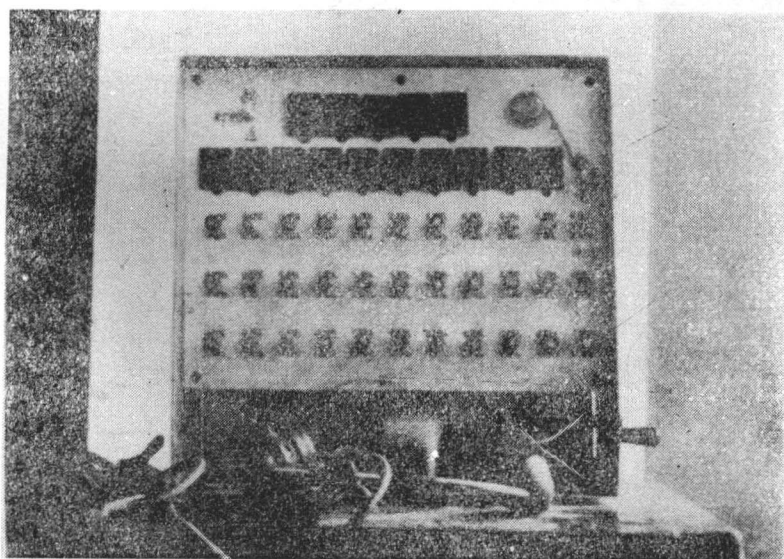
⑦ ↑ 五门自制携带式磁石交换机（60年代战备用）
