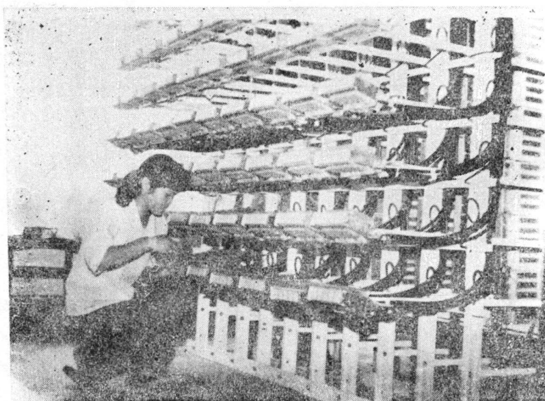
⑭ ↑ 4000门自动电话交换机配线架（八十年代使用）
