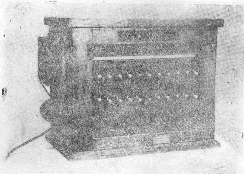
⑧ ↑10门磁石交换机（1949年末使用）
