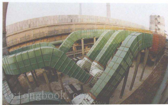
280KA槽铝电解净化系统
