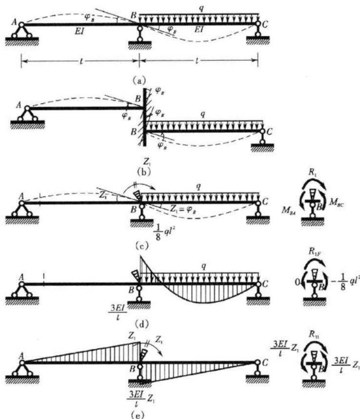
图 9-1 位移法计算连续梁
