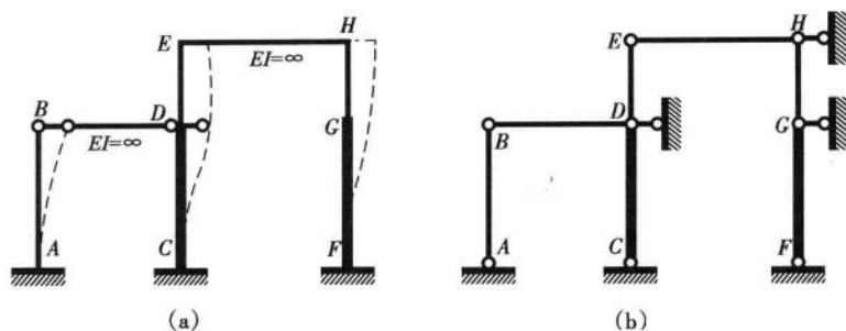
图 9-9 确定独立的结点位移数
