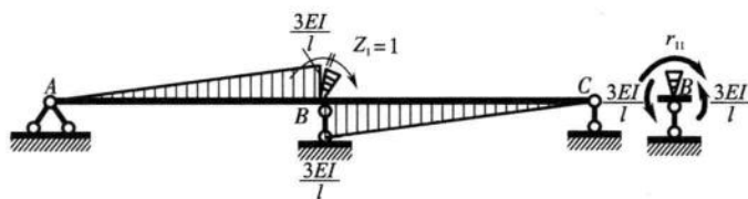
图 9-2 附加刚臂上反力偶的计算
