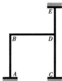
图 9-14 计算刚架结点位移数
