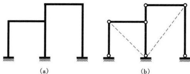
图 9-6 确定独立的结点位移数
