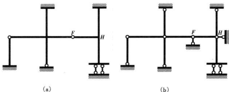
图 9-8 确定独立的结点位移数
