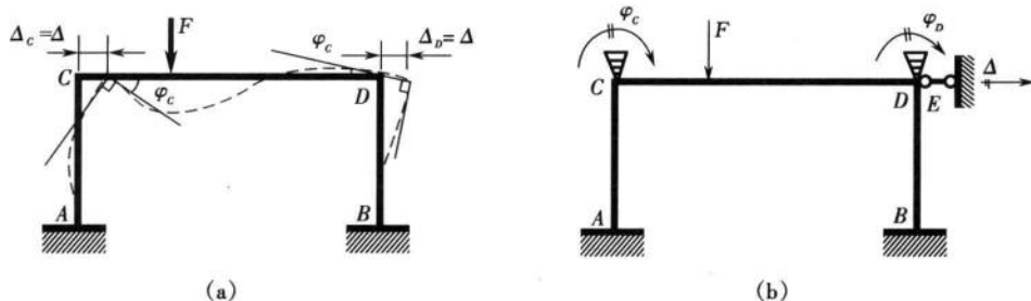
图 9-4 位移法分析刚架结构
