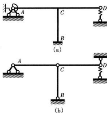
图 9-12 具有弹簧支承的结点位移数
