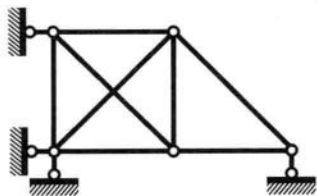
图 9-13 计算桁架结点位移数
