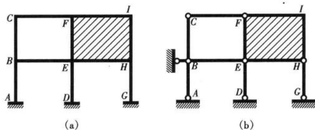
图 9-10 确定独立的结点位移数
