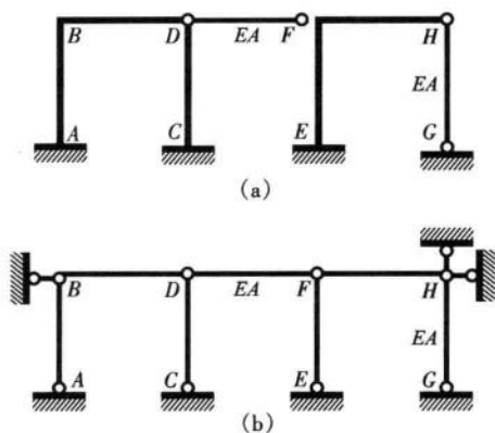
图 9-11 考虑链杆轴向变形的结点线位移
