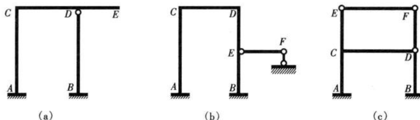
图 9-5 不作为基本未知量的结点位移
