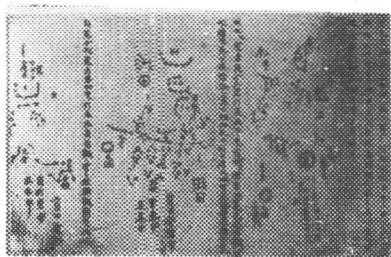
唐代敦煌星图
