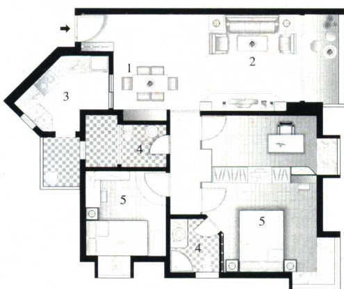
平面图
