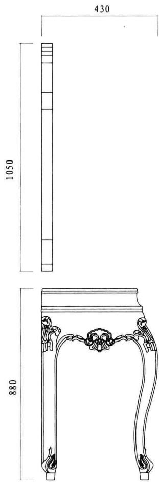
左视图
