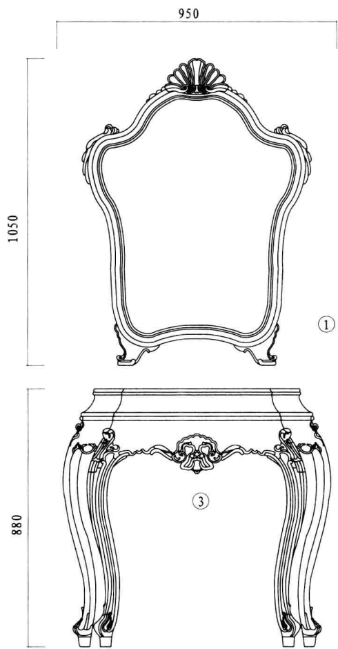
主视图
