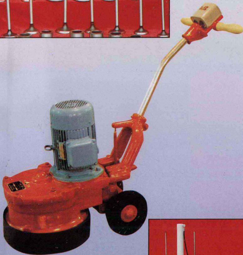
中原机械厂生产的 HMP-4 平面磨石机曾获国家建设部优 质产品奖。
