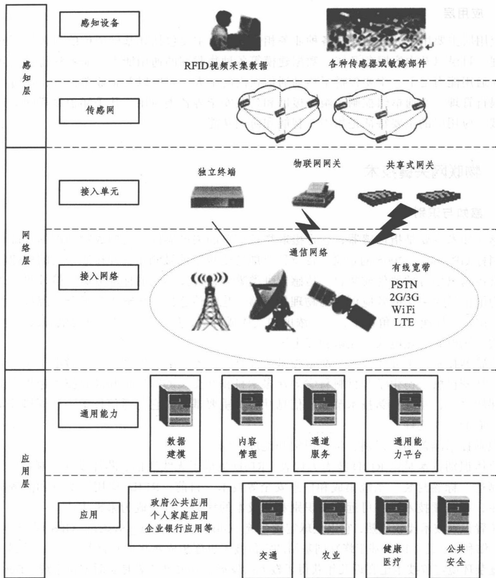
图 1.11 物联网的总体构架
