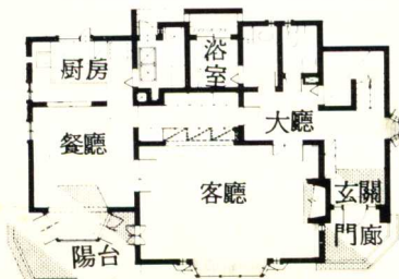
1樓平面圖
