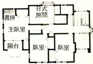
2樓平面圖
