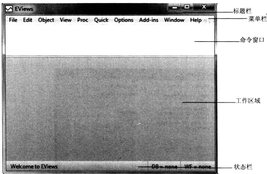
图 1-2 EViews 主窗口
