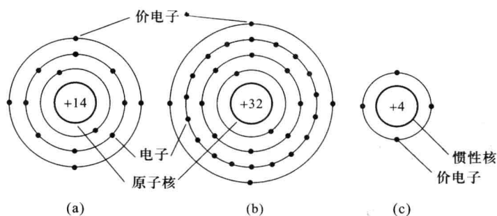
图 1.1.1 硅和锗原子结构模型
