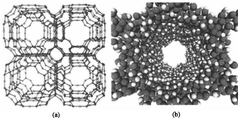
图 1.1 微孔 A 型沸石(a)和介孔 MCM-41(b)结构的比较
