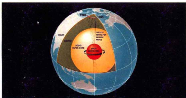
地磁场产生的“发电机原理”图示
