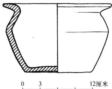
图一七 M8出土陶盆(M8:1)
