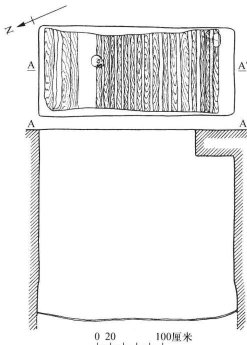
图一六 M8槨盖板平、剖面图
