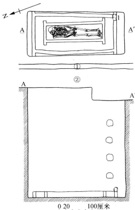
图一四 M8 平、剖面图
