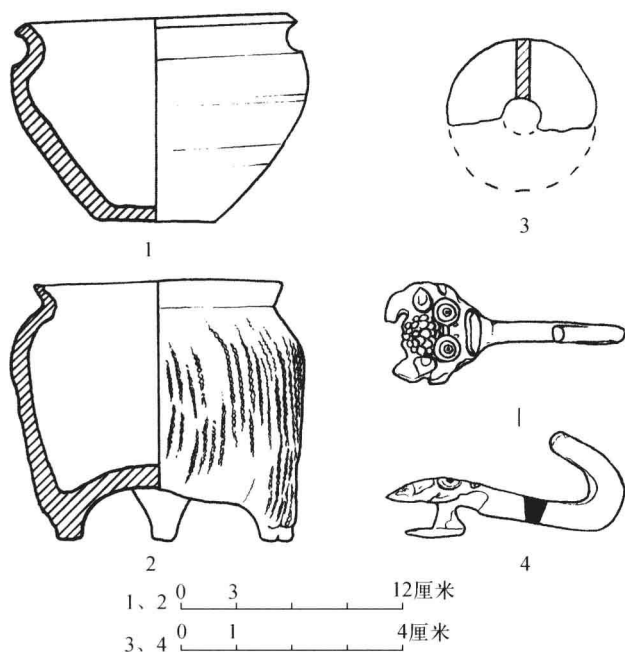
图八 M6出土器物
