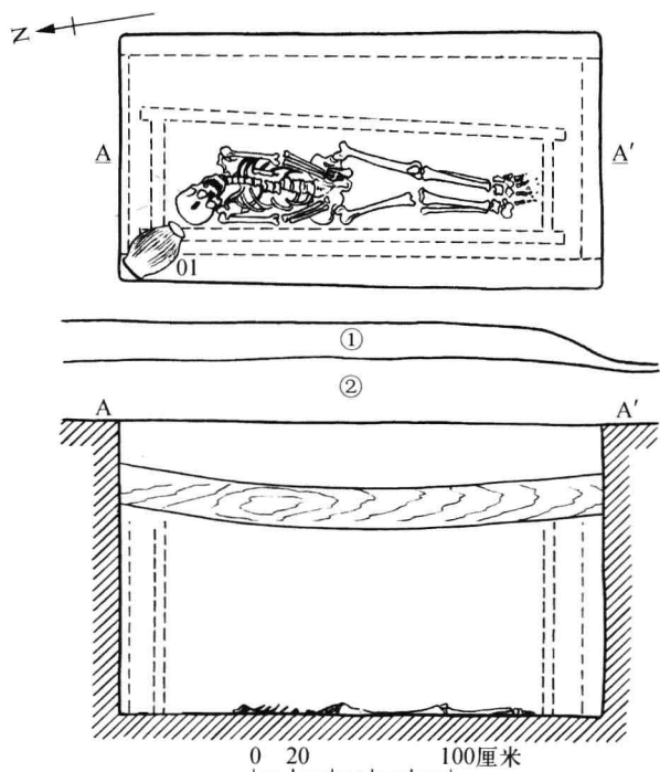
图四 M4平、剖面图
