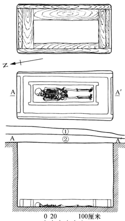
图六 M5平、剖面图
