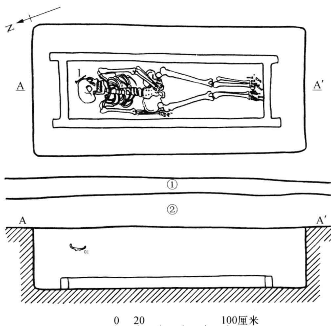
图一— M7 平、剖面图
