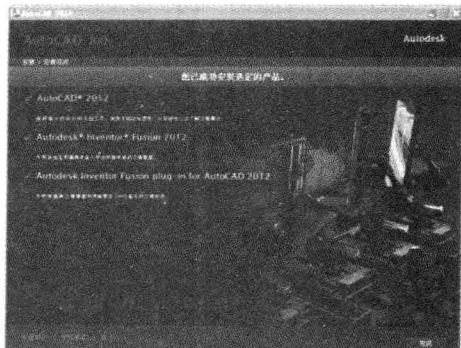
图 2-7 完成安装
