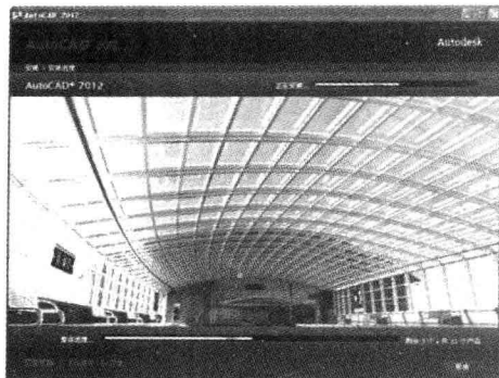
图 2-6 等待安装
