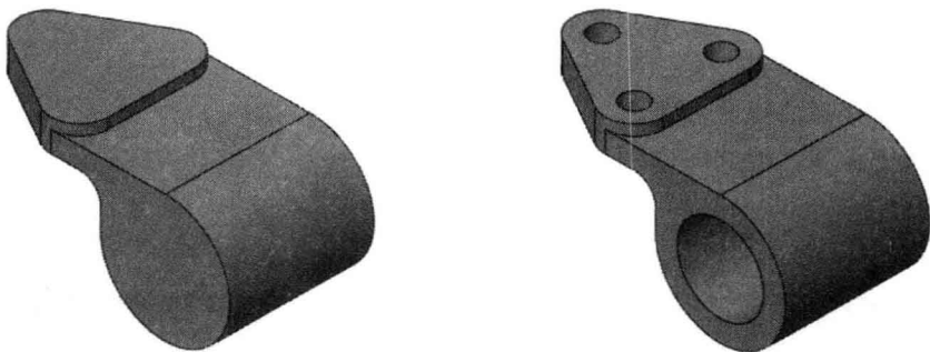
图 1-4 边线
