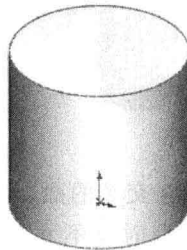
图 1-12 结果
