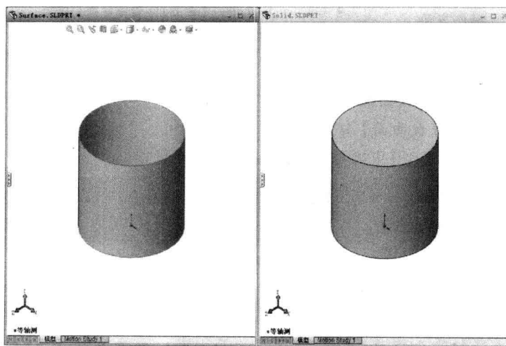
图 1-7 纵向平铺
