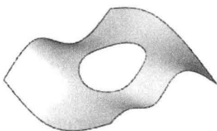
图 1-2 曲面示例
