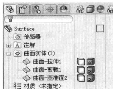
图 1-15 显示窗格
