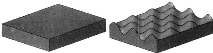
图 1-1 两个实体
