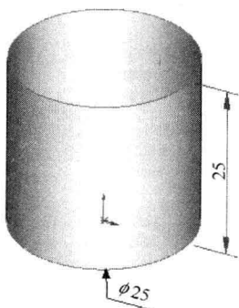
图 1-6 拉伸曲面
