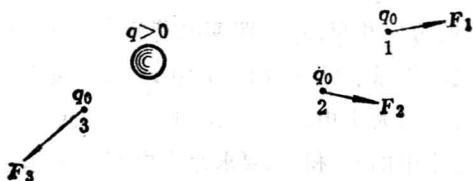
图1-2 静电荷周围的电场
