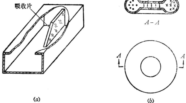
图1 微波电路中的元件
