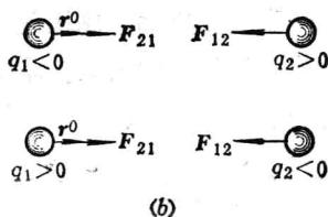
图1-1 点电荷间的作用力
