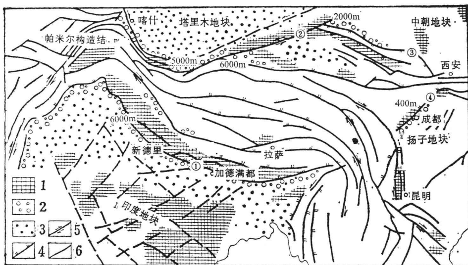
图 1-1 青藏高原构造略图
