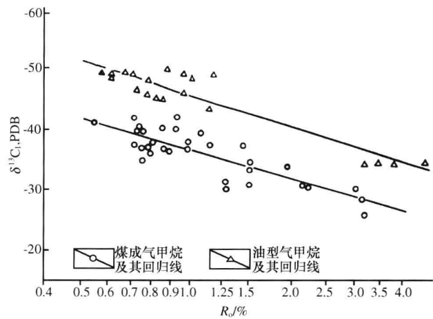
图 1 我国煤成气和油型气 \delta^{13}C_1 值与 R_a 关系图
