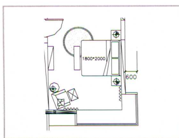
● 卧房布置图
