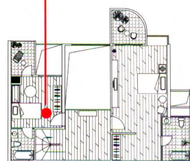
● 图1平面布置图
