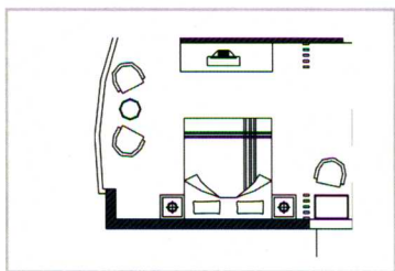
● 卧房布置图
