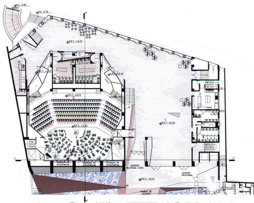
平面图 1
