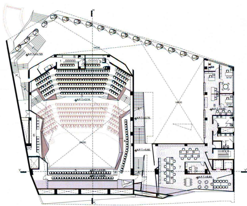
PLANTA PRIMER NIVEL FIRST LEVEL PLAN
