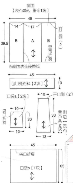
尺寸图
