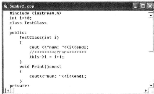
图 1-11 编辑窗口
