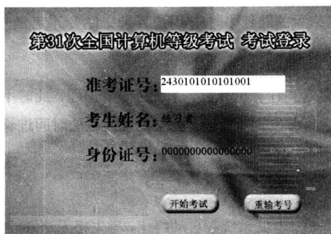
图 1-2 身份验证
