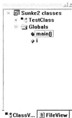
图 1-10 工作区
