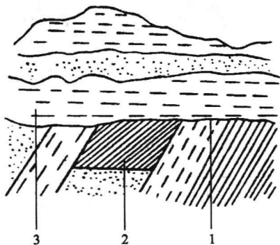
图 1-4 不整合封闭油气藏
