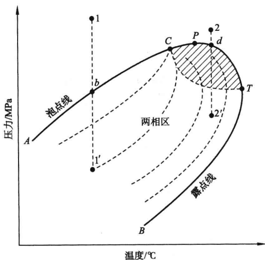
图 2-2 多组分烃类系统相图
