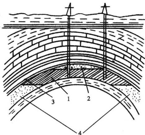
图 1-1 背斜构造油气藏
