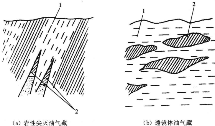
图 1-3 岩性油气藏
