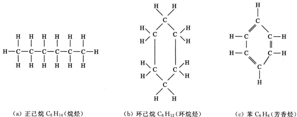
图 2-1 三种烃族的分子结构式
