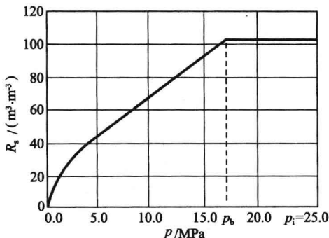
图 2-3 典型地层油一次脱气溶解气油比曲线
