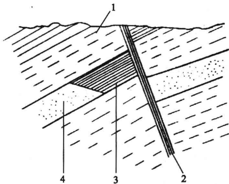
图 1-2 断层遮挡油气藏
