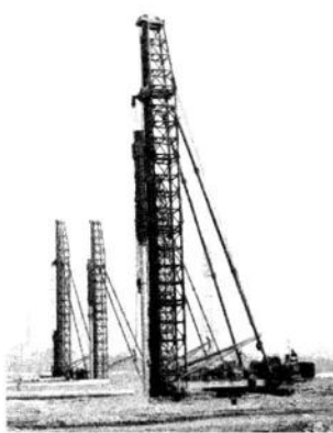
图 1.12 锤击沉桩法
