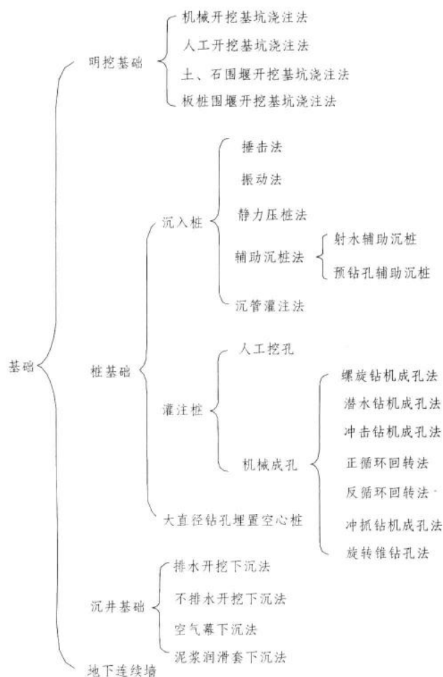
图 1.10 桥梁基础分类及施工方法
