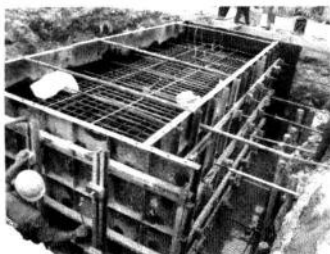
图 1.18 旱地承台施工
