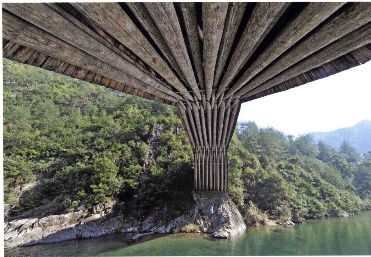
木拱桥架底部仰视
