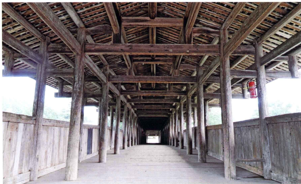
桥屋
