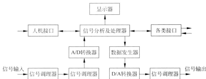
图 1-1 虚拟仪器的结构
