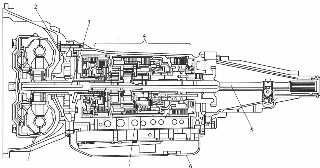
图 1-2 前置后驱自动变速器
