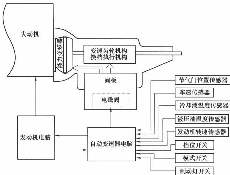
图 1-4 电控液力自动变速器控制原理图
