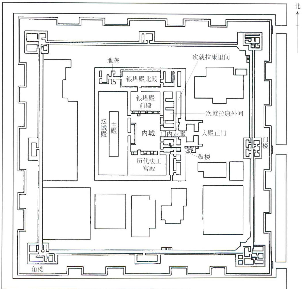
图 2-2 萨迦寺平面布局示意图
