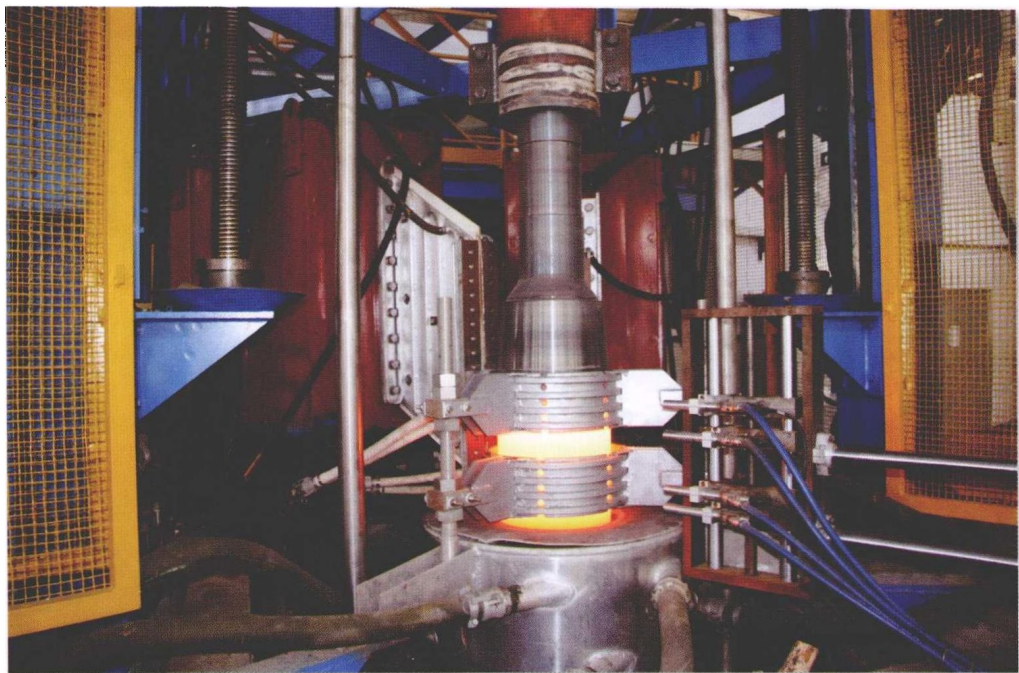
双频淬火机床
