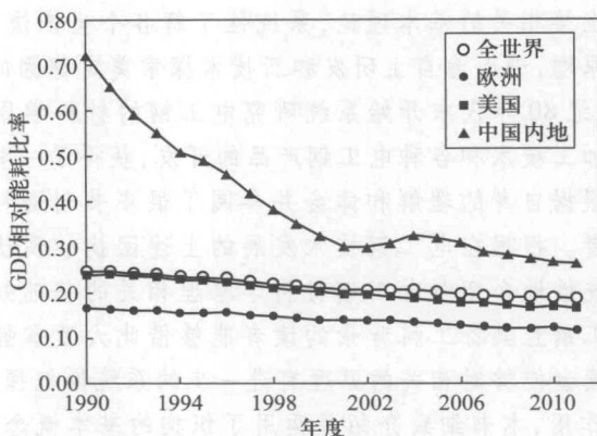
图 0.3 GDP 相对能耗比率参数的变化 (Enerdata 能源资讯公司)
