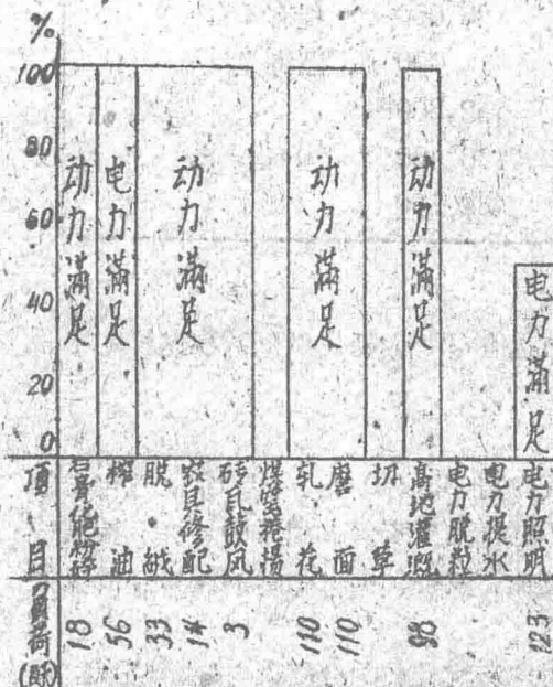
图 1. 曲亭1959年负荷水平及负荷表
