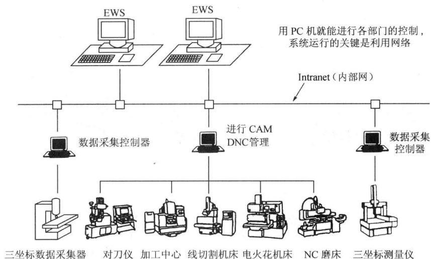
图 1.4 CAD/CAM 硬件组成示例
