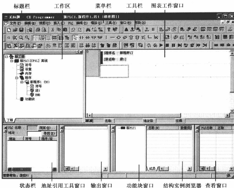
图 1-1 CX-Programmer 编程软件界面
