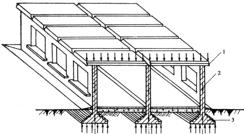
图 1-1 建筑物荷载传递示意图
