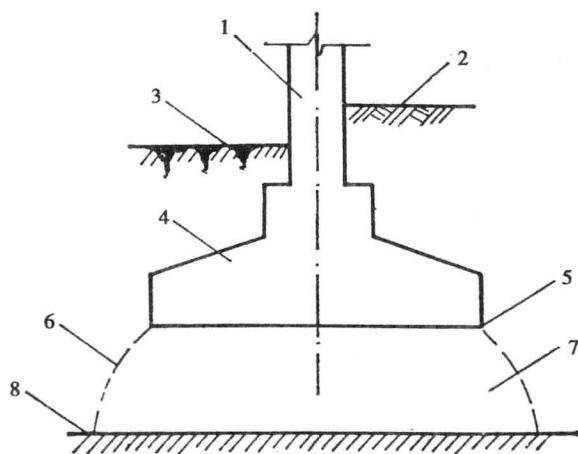
图 1-2 地基基础示意图
