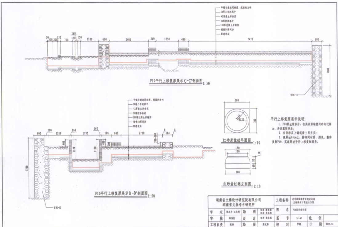
图版六 永顺老司城遗址F10回填保护剖面图
