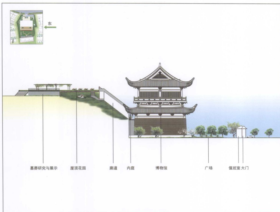
图版二 桂阳刘家岭壁画墓博物馆竖向示意图
