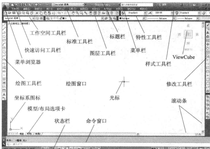
图 2-3 AutoCAD 2013 的经典工作界面
