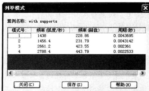
图1-7 列举模式
