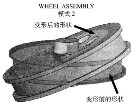
图 1-2 车轮变形前后的形状对比
