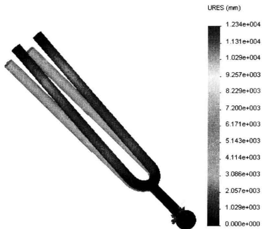
图 1-9 音叉变形前后的位置对比
