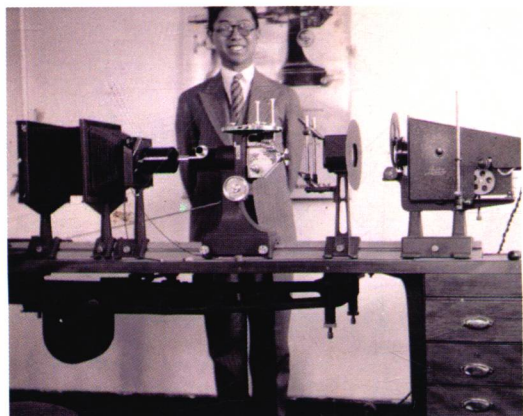
张维在唐山交大工作期间做光弹性实验
