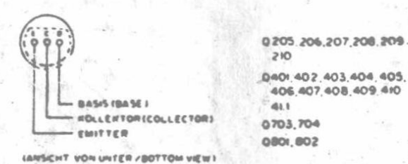
晶体管与集成电路引线图
