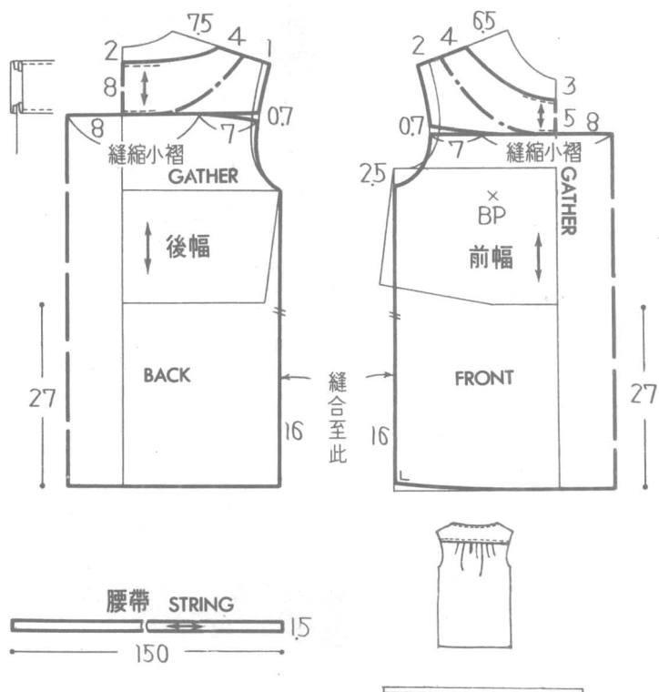
展開圖
