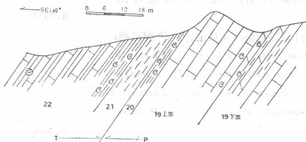
图 1—3 四川广元上寺长江沟剖面二叠—三叠系界线素描图
