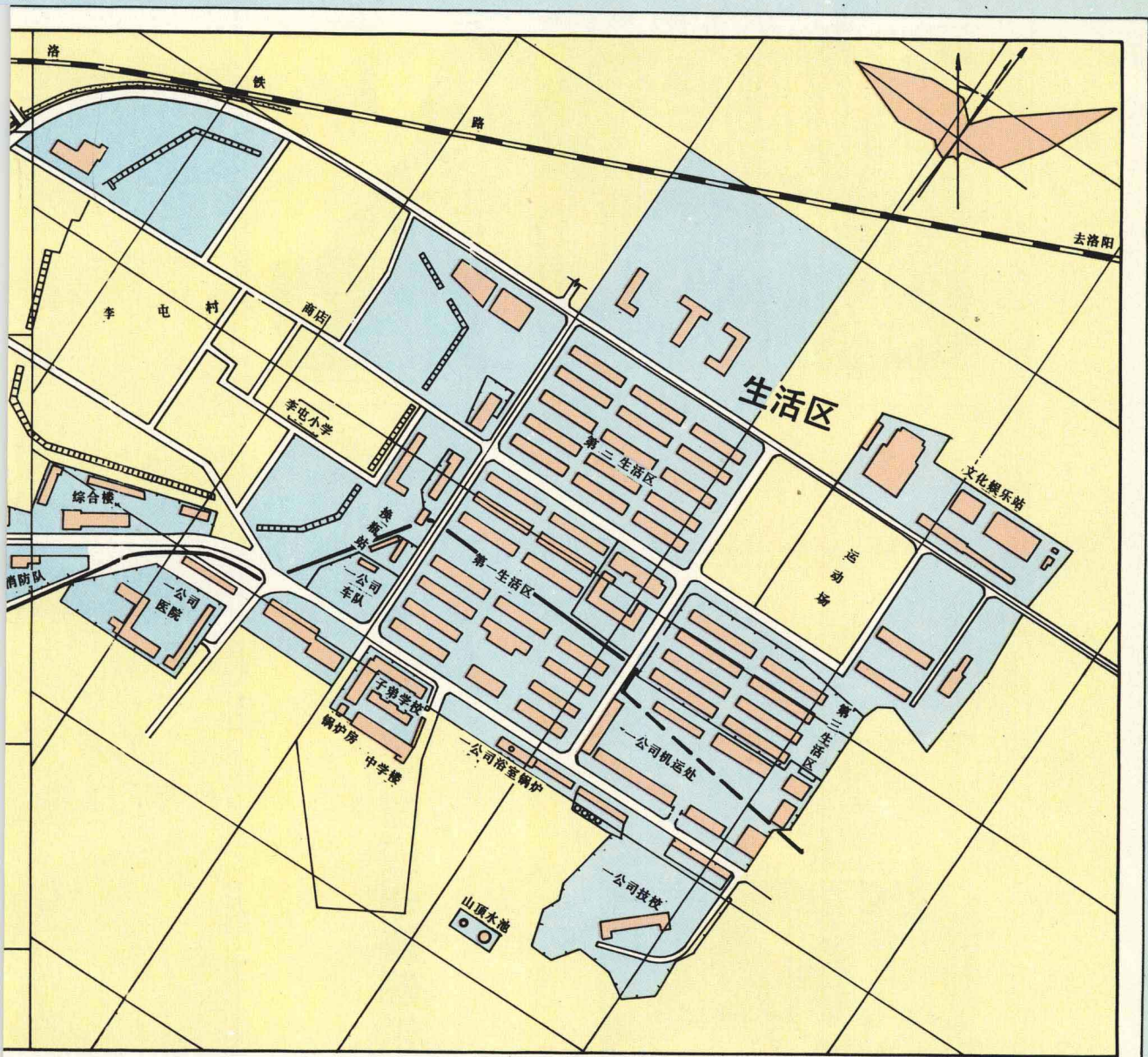
工程公司李屯基地总平面图
